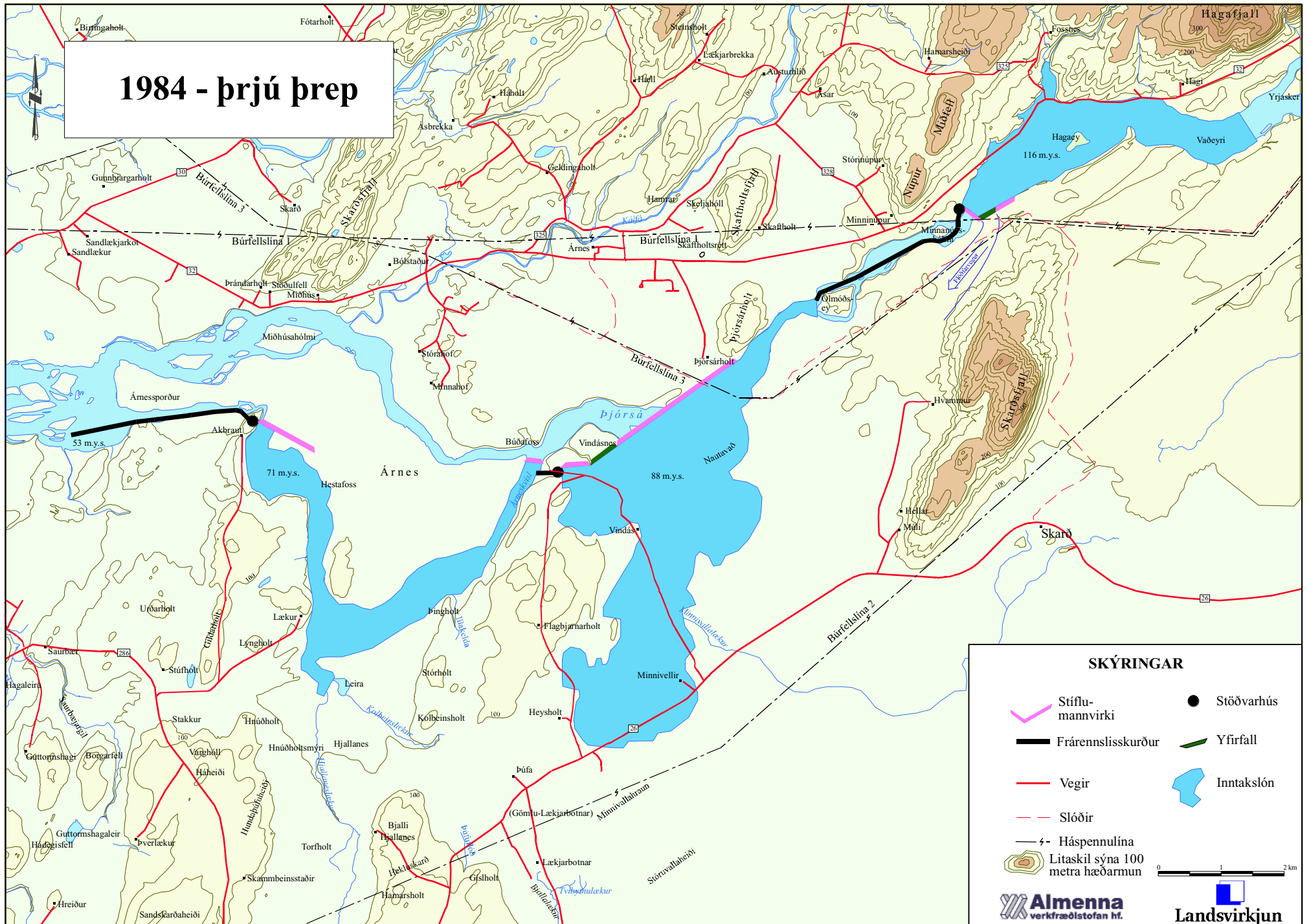
8. mynd. Hugmynd Verkfræðistofu Sigurðar Thoroddsen hf. frá 1984 um virkjun fallsins í Björnsá frá Núpi niður fyrir Arnessporð í þremur áföngum. Utlínur lóna eru byggðar á gömlum og tiltölulega ónákvæmum kortum
